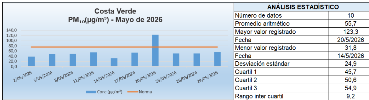
Gráfico 5: Análisis estadístico estación Costa Verde, mayo de 2026.
