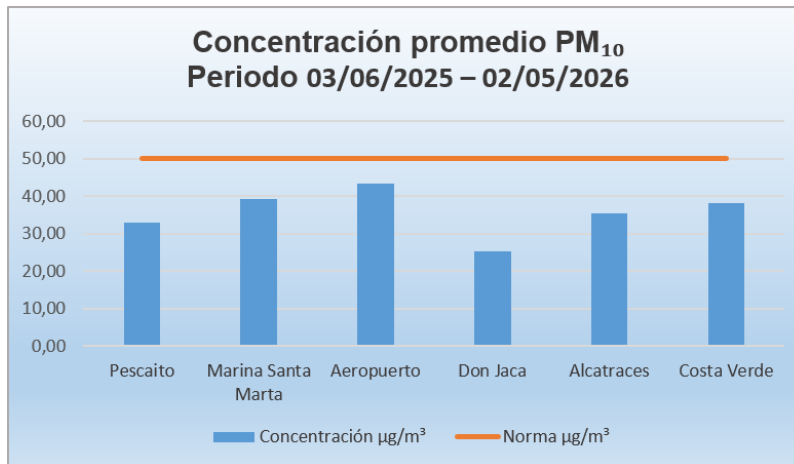
Gráfico 9: Promedio registrado en las estaciones de monitoreo PM 10 , 03/06/2025 – 02/05/2026.
