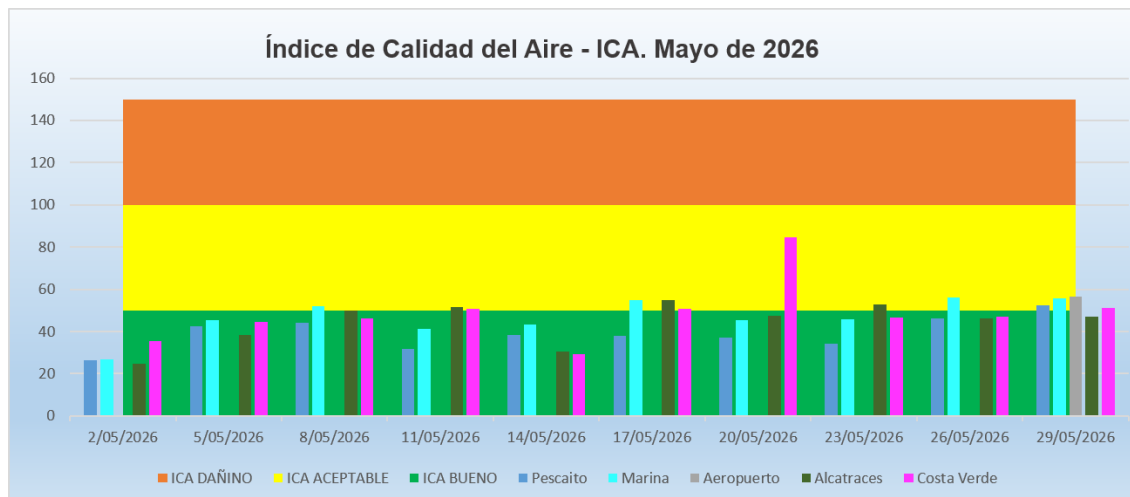
Gráfico 10: Índice de Calidad del Aire, perfil de los valores estimados, mayo de 2026.
