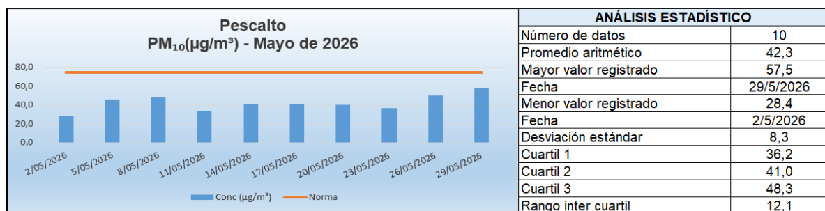
Gráfico 1: Análisis estadístico estación Pescaito, mayo de 2026.
