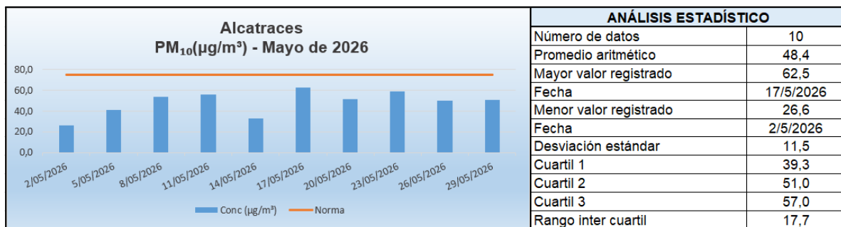
Gráfico 4: Análisis estadístico estación Alcatraces, mayo de 2026.
