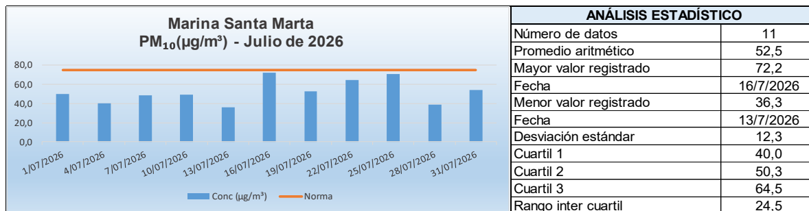
Gráfico 2: Análisis estadístico estación Marina Santa Marta, julio de 2026.
