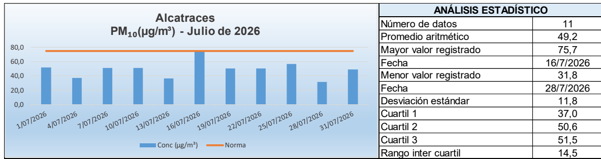
Gráfico 4: Análisis estadístico estación Alcatraces, julio de 2026.
