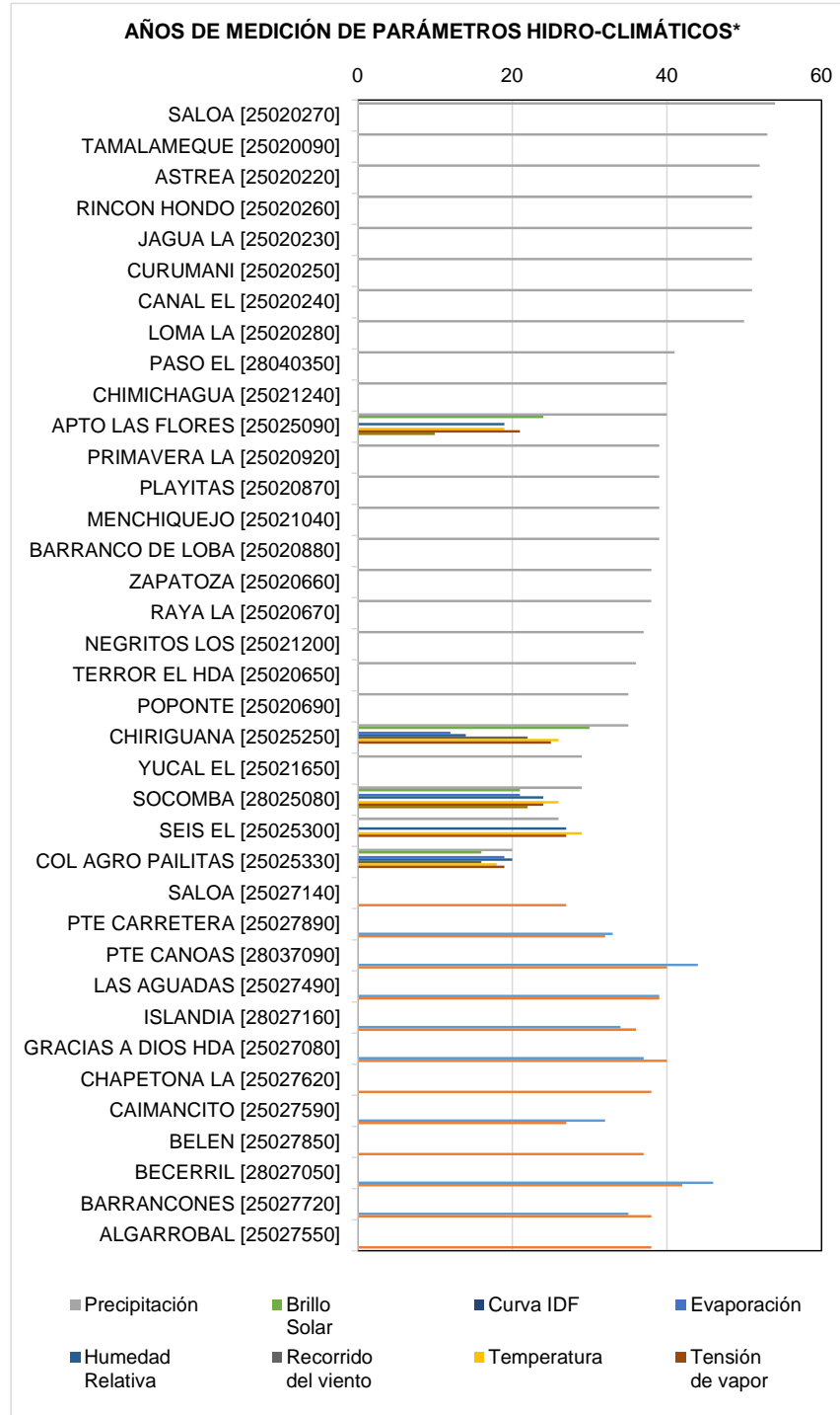
Figura 5.10. Años de medición de parámetros hidro-meteorológicos.
