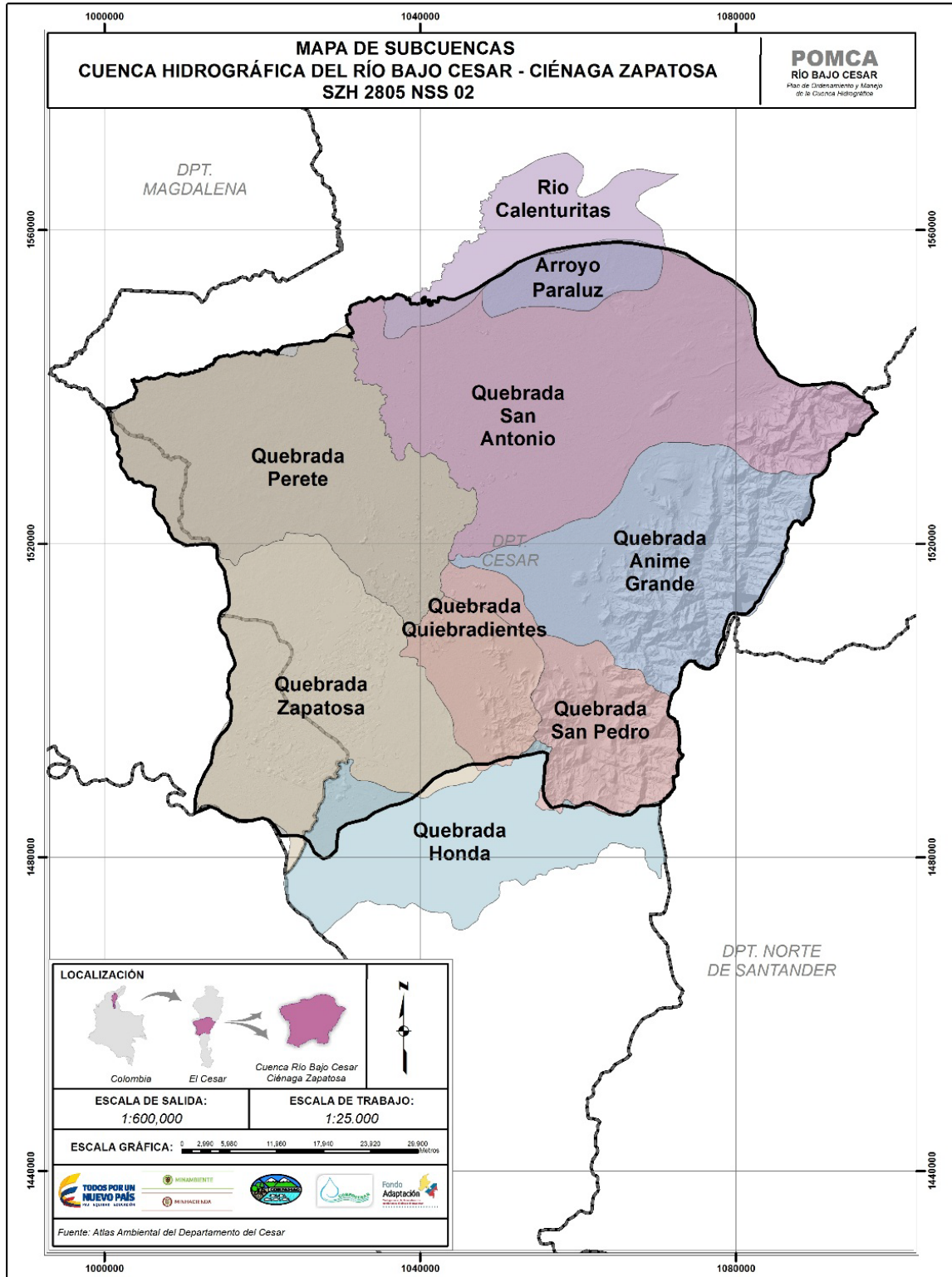
Figura 6.11. Mapa de subcuencas Bajo Cesar – Ciénaga Zapatosa.
