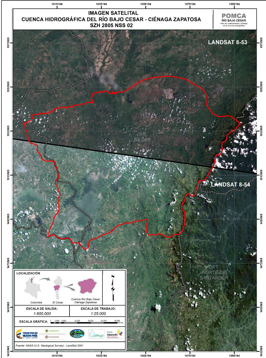
Figura 5.8. Imagen LANDSAT 8-53, 8-54.
