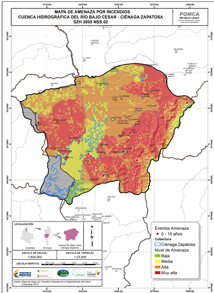
Figura 6.106. Mapa de amenaza por incendios forestales.
