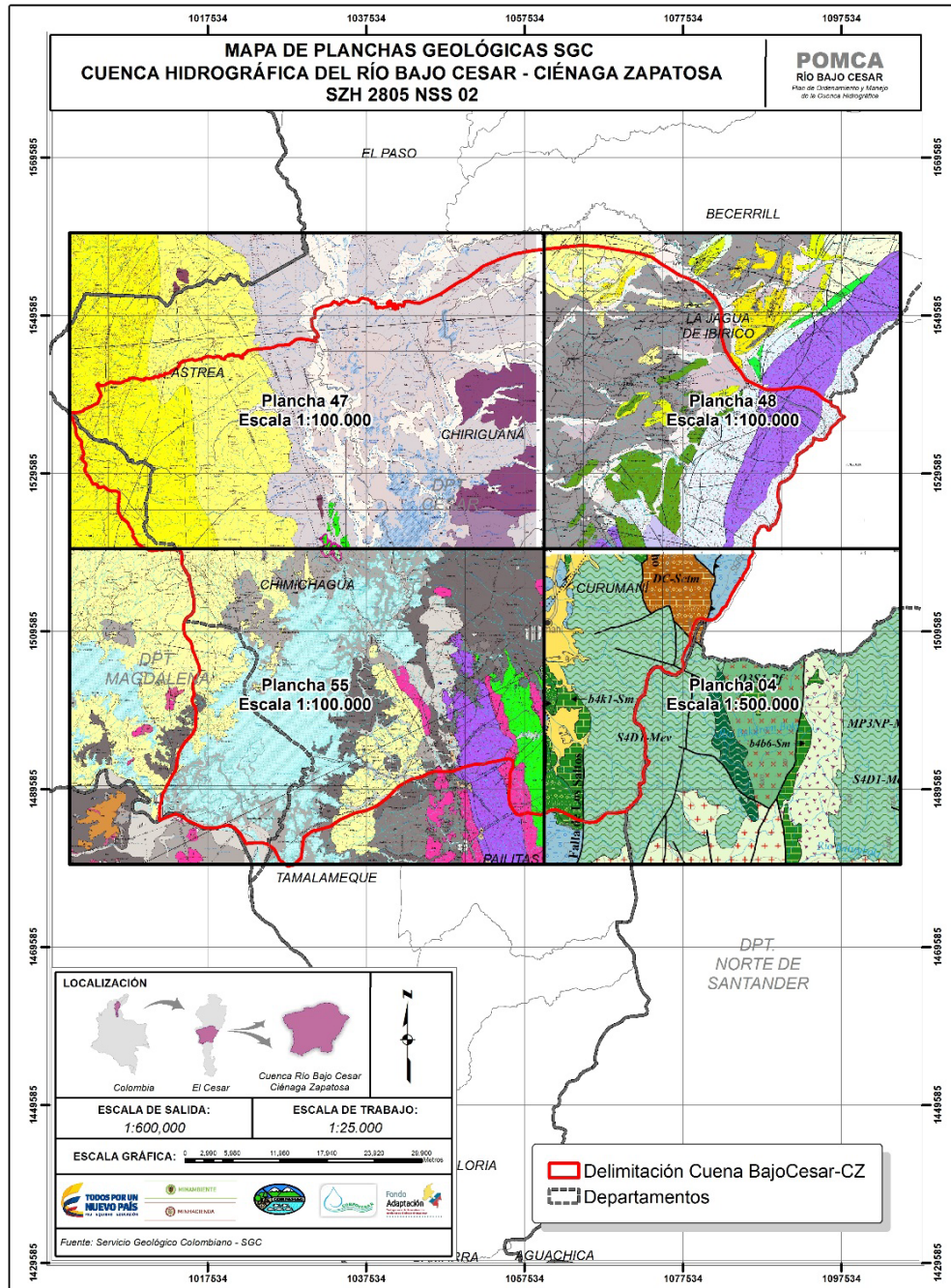
Figura 5.11. Planchas geológicas.
