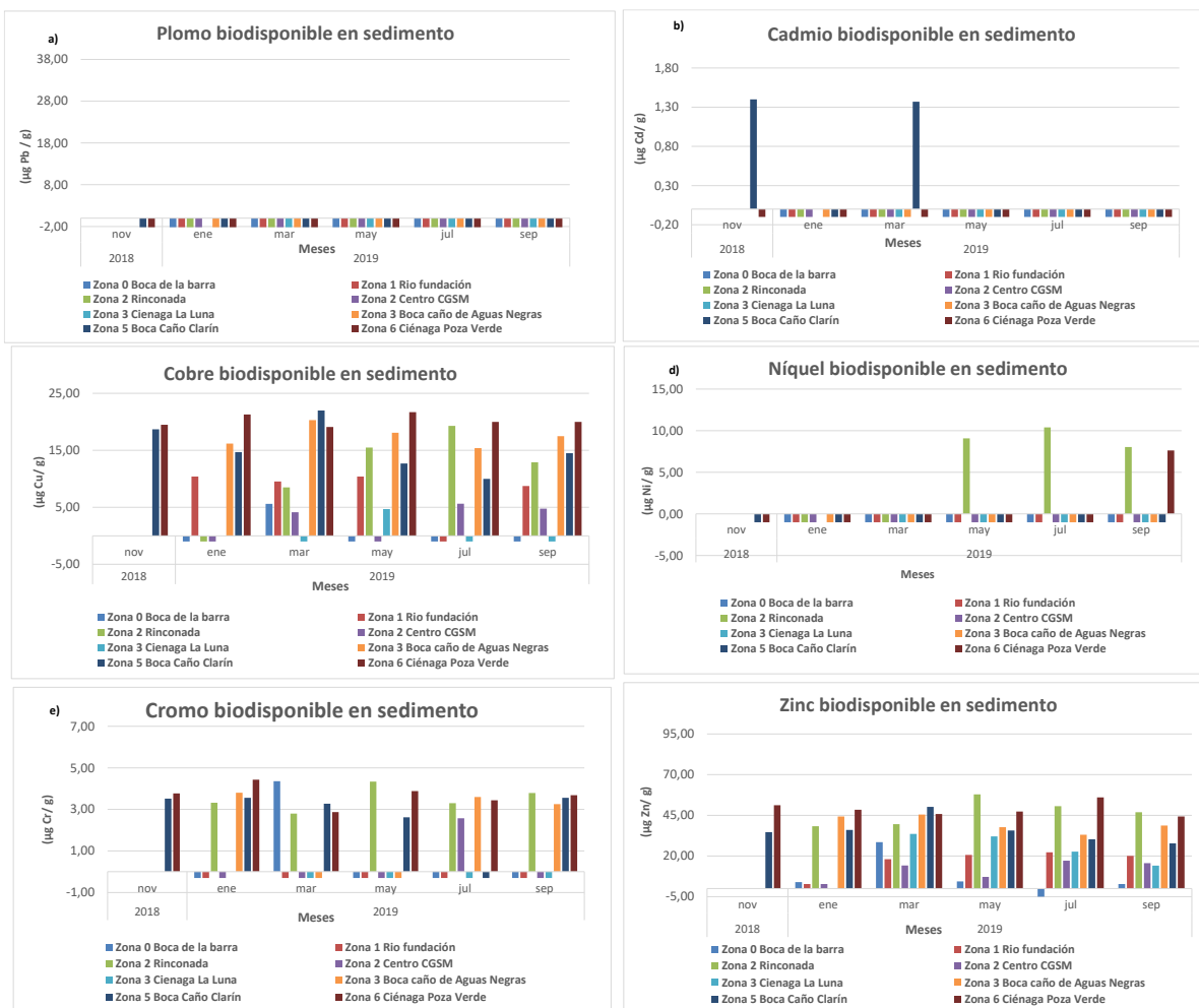
Figura 4.1-36. Concentración biodisponible de a) Plomo (Pb), b) Cadmio (Cd), c) Cobre (Cu), d) Níquel (Ni), e) Cromo (Cr), f) Zinc (Zn) en sedimentos de las seis zonas de monitoreo de la Ciénaga Grande de Santa Marta medidos entre noviembre del 2018 y septiembre del 2019. Barras por debajo de cero representan valores menores al límite de cuantificación de la técnica analítica.
