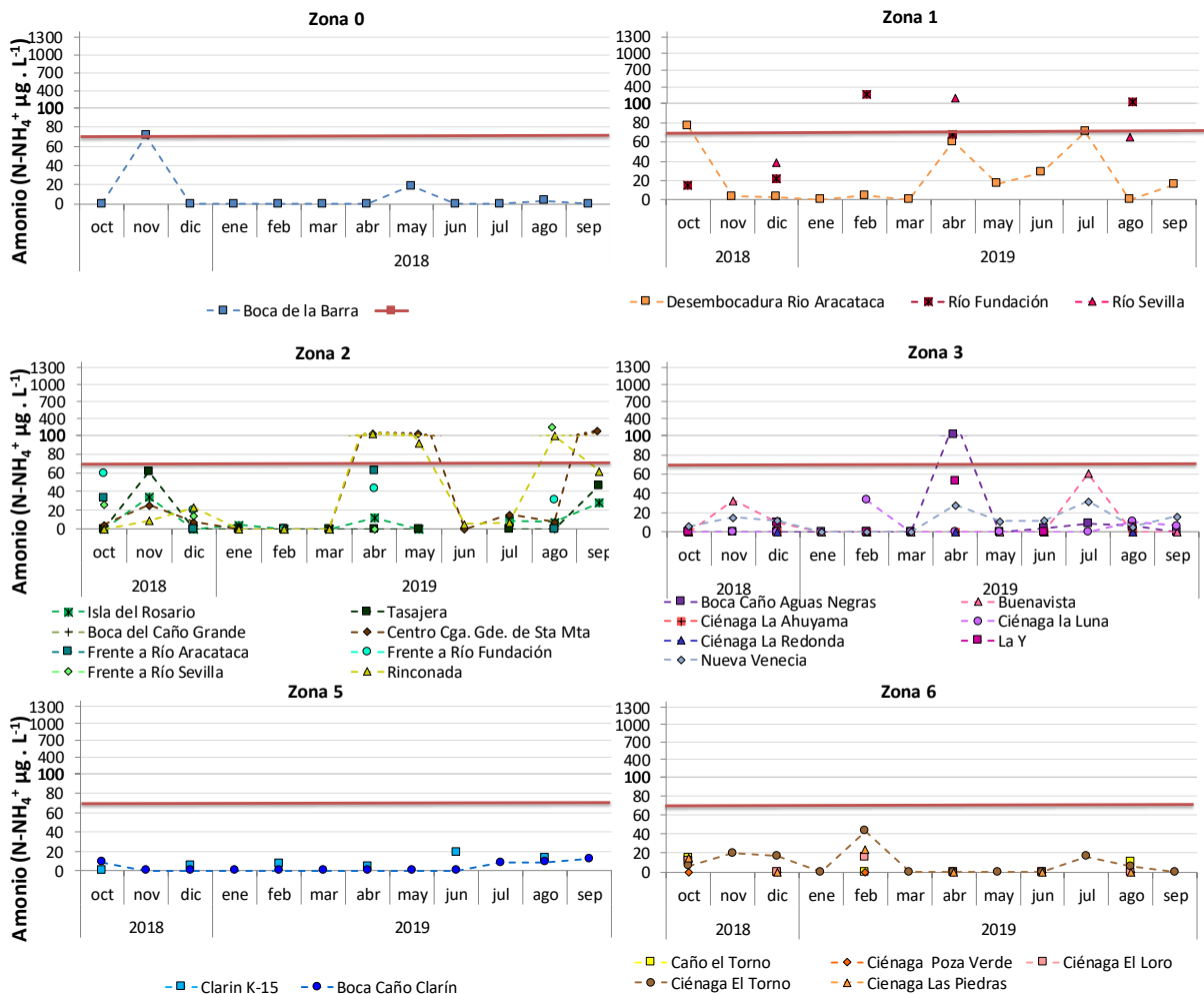
Figura 4.1-17. Concentraciones de Amonio ( \mu\text{g N-NH}_4^+/\text{L} ) en el agua superficial de las seis zonas de la CGSM, durante el monitoreo octubre de 2018 - septiembre de 2019. Línea horizontal roja representa el valor considerado típico en estuarios poco contaminados (70,0); (Fraile et al. , 1991).
