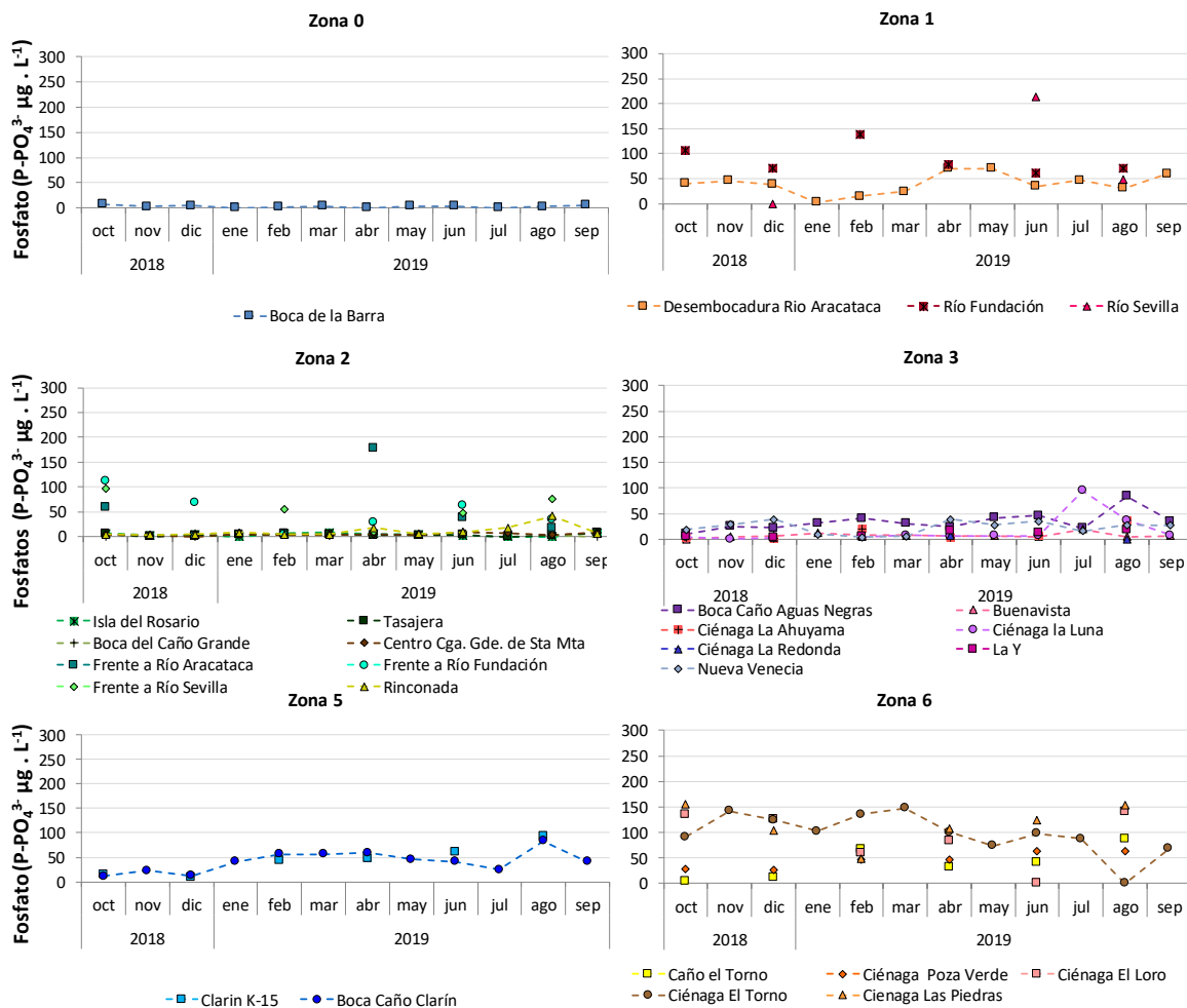
Figura 4.1-21. Concentraciones de Fosfatos ( \mu\text{g P-PO}_4^{3-}/\text{L} ) en el agua superficial de las seis zonas de la CGSM, durante el monitoreo octubre de 2018-septiembre de 2019.
