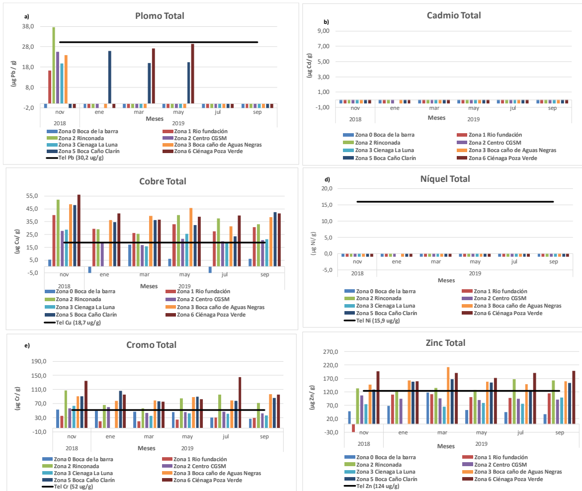
Figura 4.1-32. Concentración total de a) Plomo (Pb), b) Cadmio (Cd), c) Cobre (Cu), d) Níquel (Ni), e) Cromo (Cr), f) Zinc (Zn) en sedimentos de las seis zonas de monitoreo de la Ciénega grande de Santa Marta medidos entre noviembre del 2018 y septiembre del 2019, comparados con el nivel umbral de efectos – TEL (Threshold Effect Level) – establecido en las tablas SquiRTs de la NOAA (Buchman, 2008). Barras por debajo de cero representan valores menores al límite de cuantificación de la técnica analítica.
