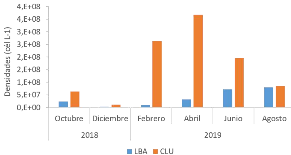
Figura 4.1-48. Valores de la densidad fitoplanctónica (cel. L -1 ) registrado en las estaciones de Boca de la Barra (LBA) y Ciénaga la Luna (CLU), entre octubre de 2018 y agosto de 2019.
