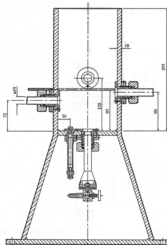
Figura 3.4. Dispositivo de calentamiento y protección - Prueba Koenen
