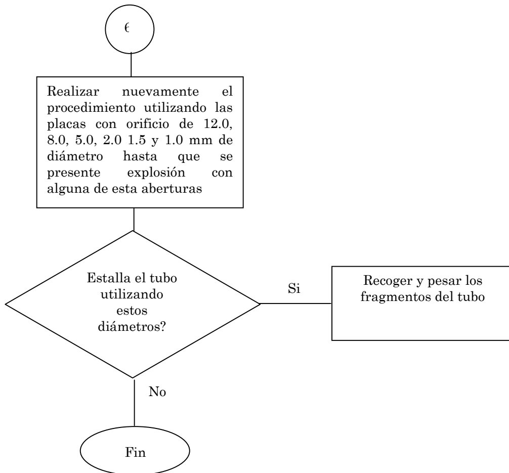
Figura 3.5. Diagrama de flujo procedimiento para determinación de la sensibilidad de sustancias ante el calentamiento en espacio limitado
