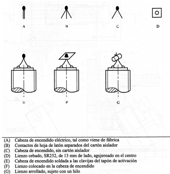
Figura 3.9. Sistema de ignición para sólidos equipo para realización de prueba tiempo/presión
