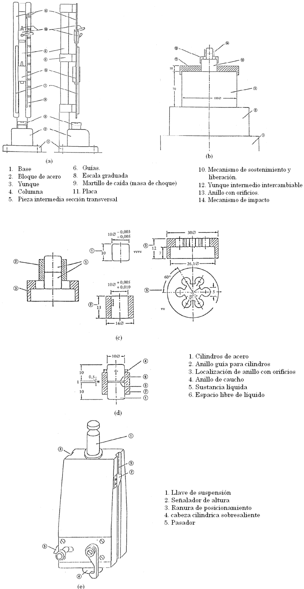
Figura 3.14. Equipo de prueba para determinación de explosividad por sensibilidad al choque. (a). Vista frontal. (b). Vista de la parte inferior del equipo. (c). Detalles mecanismo de choque para sustancias sólidas y pastosas. (d). Detalles mecanismo de choque para sustancias líquidas. (e). Detalles martillo de caída (masa de choque).
