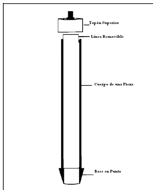
Figura X.12. Muestreador Penetrante
