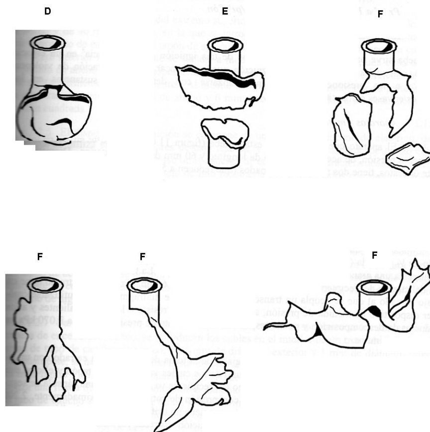
Figura 3.6. Posibles efectos en el tubo utilizado en el procedimiento - Prueba Koenen
