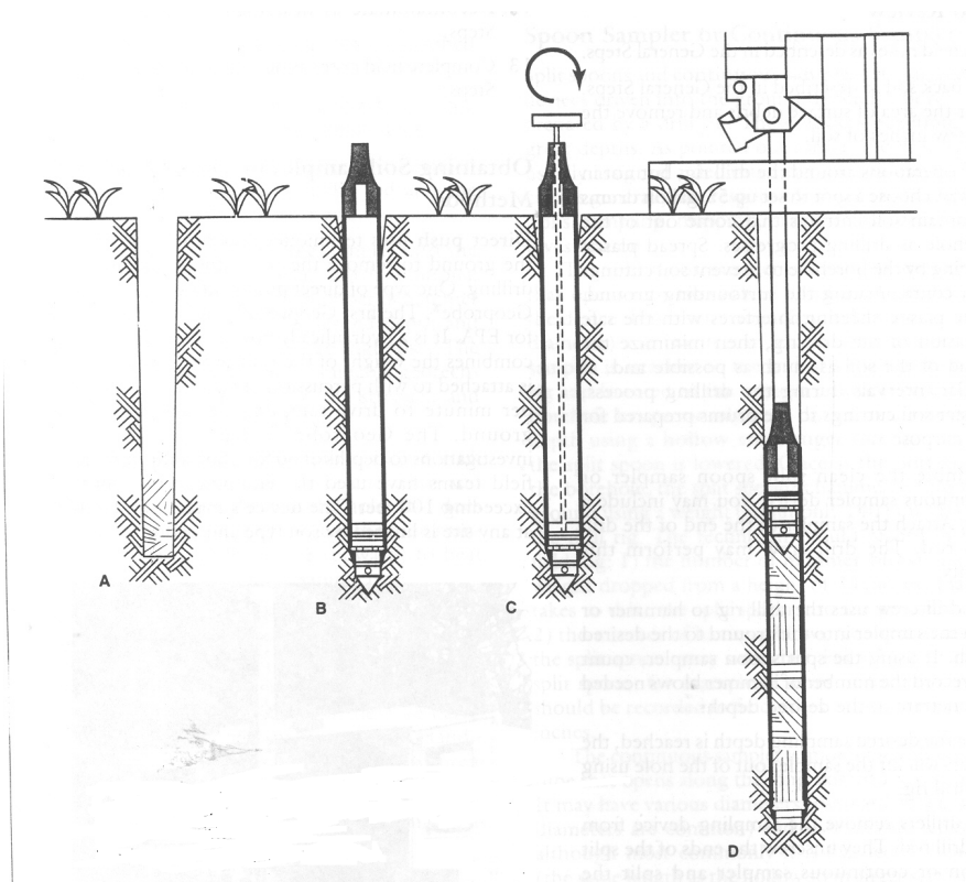
Figura 1.7. Diferentes taladros usados para diferentes tipos de suelos
