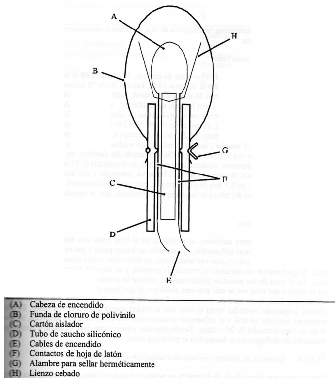
Figura 3.10. Sistema de ignición para líquidos equipo para realización de prueba tiempo/presión
