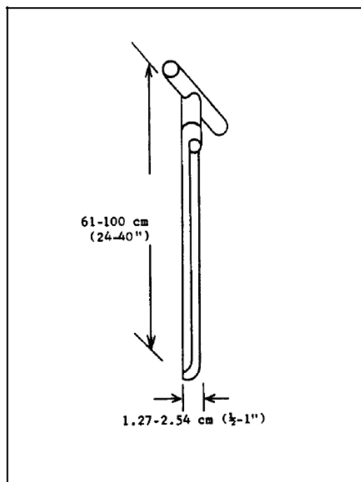
Figura X.15. Traer
