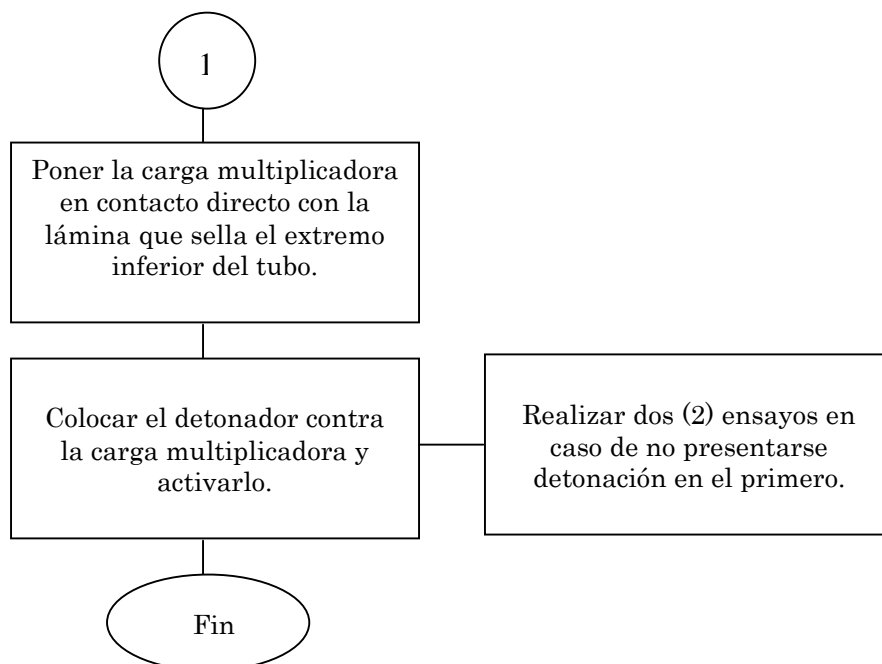
Figura 3.2. Diagrama de flujo procedimiento para determinación de sustancias que tienen la capacidad de propagar la detonación.
