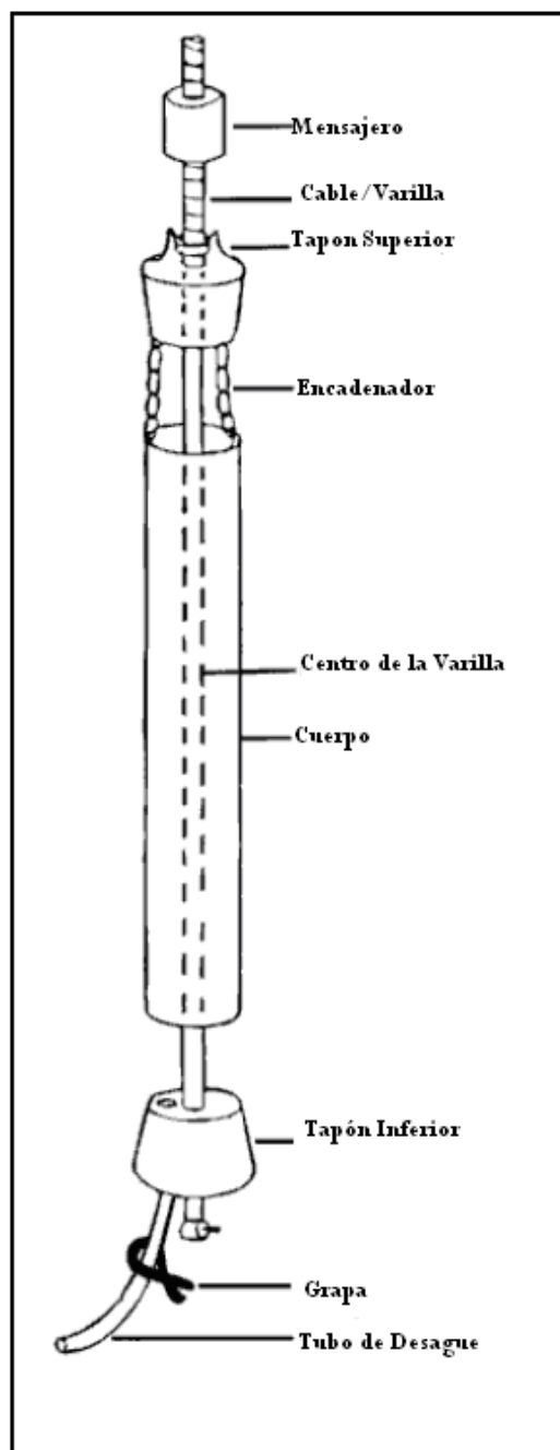
Figura X.8. Muestreador Kemmerer
