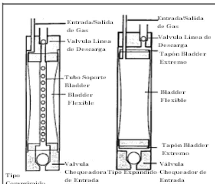
Figura X.2. Bomba Bladder
