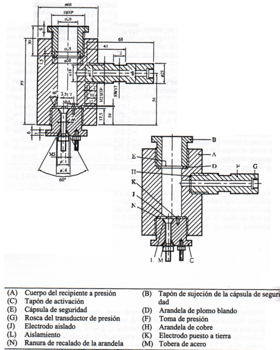
Figura 3.7. Equipo para realización de prueba tiempo/presión
