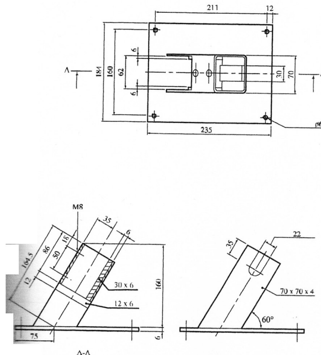
Figura 3.8. Soporte equipo para realización de prueba tiempo/presión
