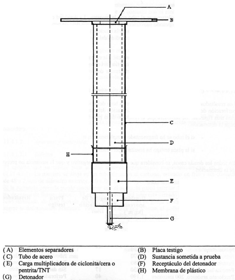
Figura 3.1. Equipo para prueba de excitación con barrera interpuesta.
