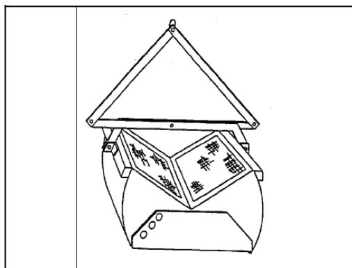
Figura X.6. Dragador Ponar
