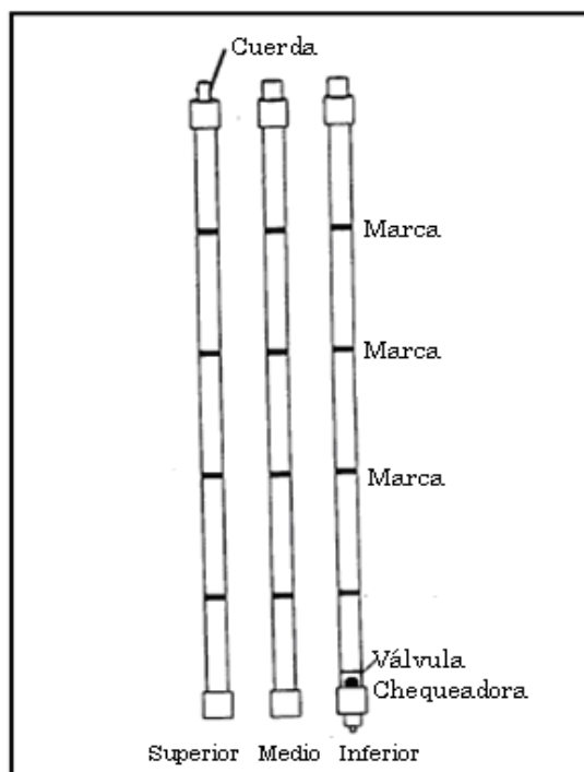
Figura X.26. Perfilador de Sólidos Fijos
