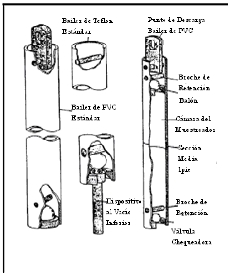
Figura X.27. Bailer
